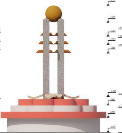
Фасад А М 1:20
