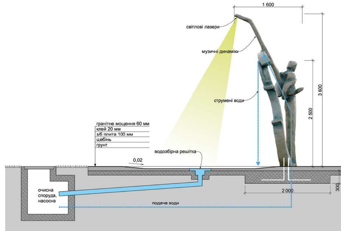
ФАСАД СКУЛЬПТУРИ З ФОНТАНОМ М 1:20
