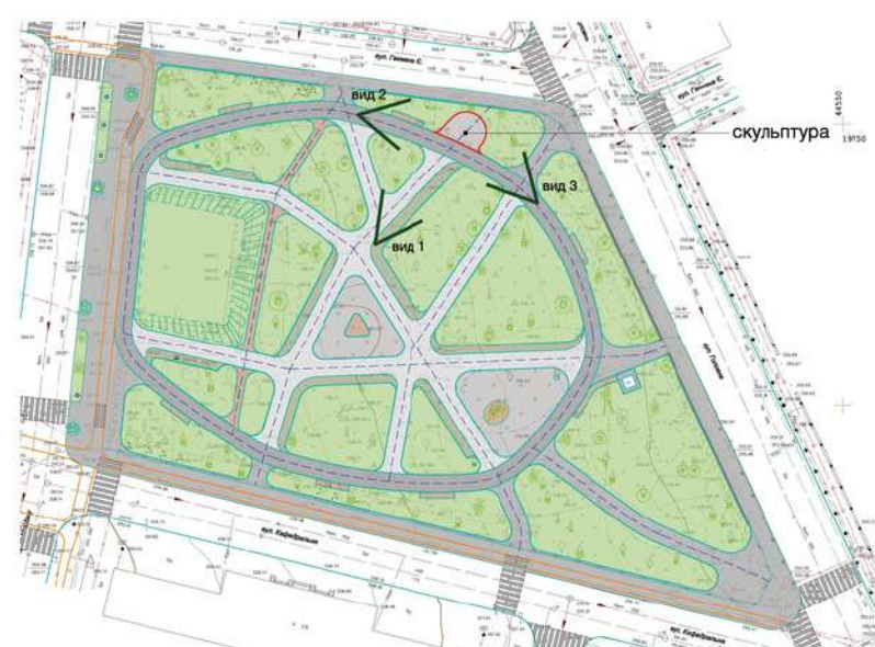
ГЕНЕРАЛЬНИЙ ПЛАН ПАРКУ М 1:500
