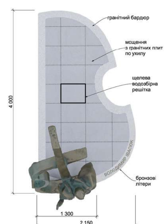
ПЛАН СКУЛЬПТУРИ З ФОНТАНОМ М 1:20
