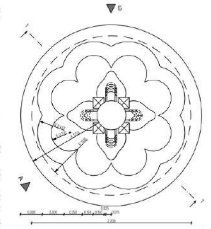
План М 1:20
