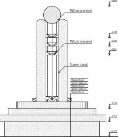
Розріз 1-1 М 1:20
