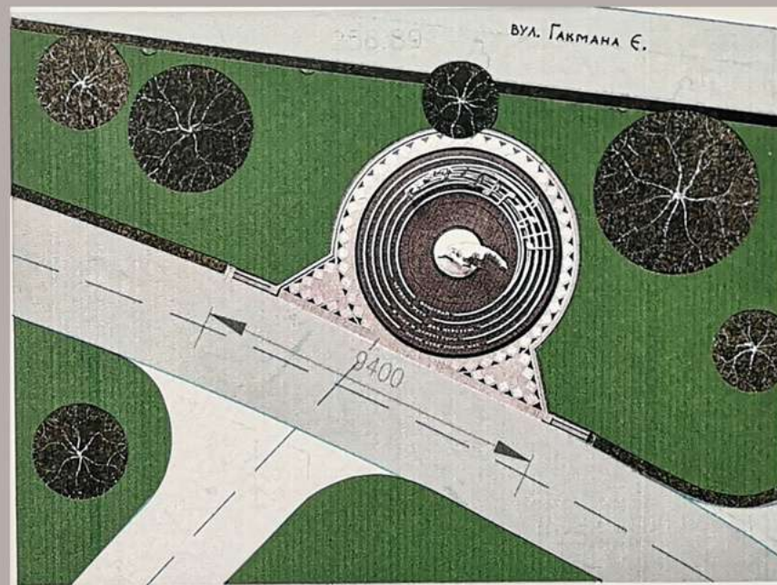
3. План з розміщенням пам'ятника
