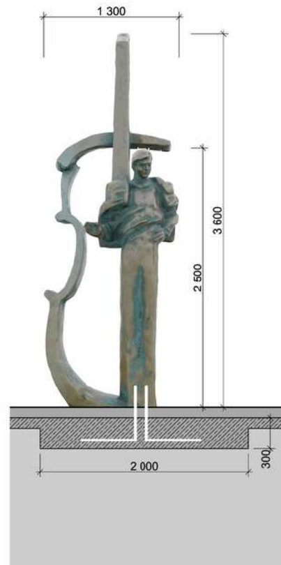
РОЗРІЗ СКУЛЬПТУРИ З ФОНТАНОМ М 1:20
